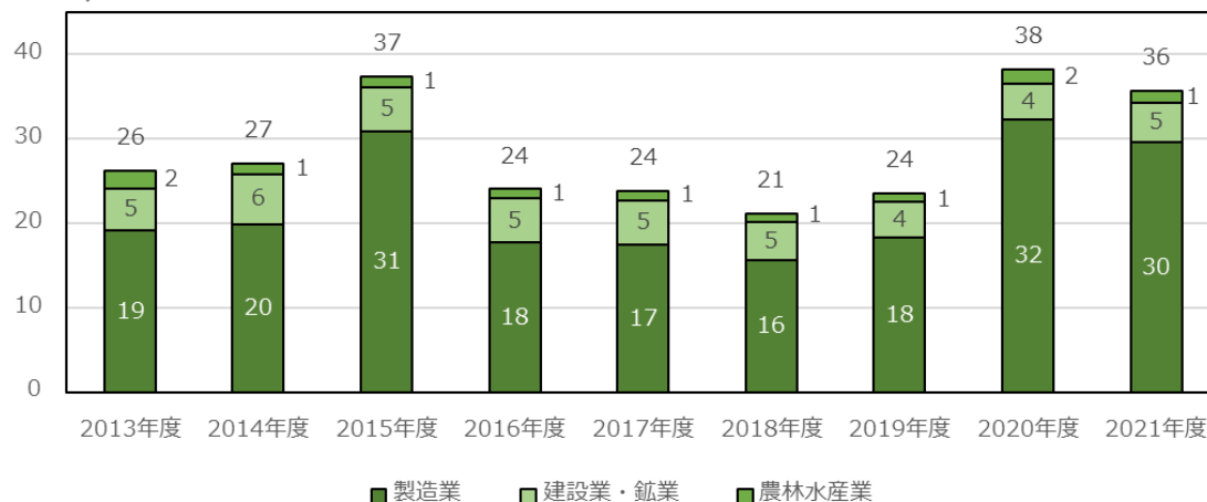
図3 産業部門におけるCO2排出量の推移
