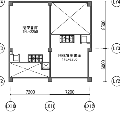
M2F平面図
